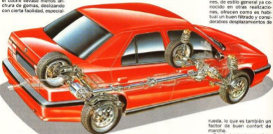
El sistema de transmisión, con acoplamiento central Ferguson y diferencial Torsen trasero, repite el esquema del Delta Integralé.
